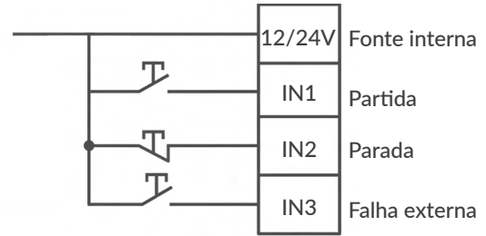
Comando a três fios
