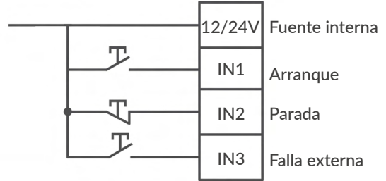
Control a tres hilos
