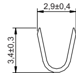
Seção B-B
