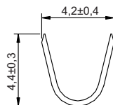
Seção A-A
