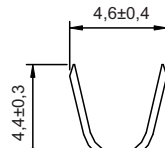
Seção A-A
