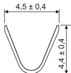
Seção B-B
