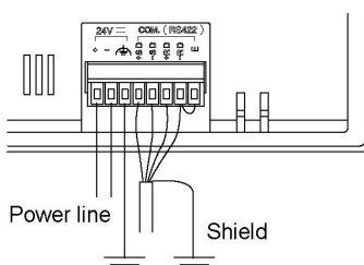
GT05/GT32/GT32-E
