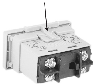
Adaptador e suporte de fixação acompanham o produto Flush adapter and mounting frame are supplied with the product
