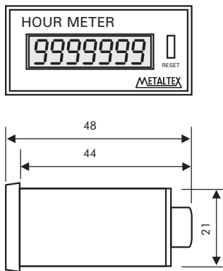
Adaptador e suporte de fixação acompanham o produto Flush adapter and mounting frame are supplied with the product
