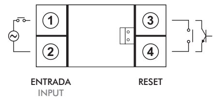
ENTRADA TENSÃO VCA AC VOLTAGE INPUT
