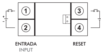
ENTRADA TENSÃO VCC DC VOLTAGE INPUT
