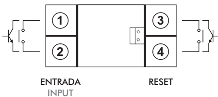
ENTRADA CONTATO NO VOLTAGE INPUT
